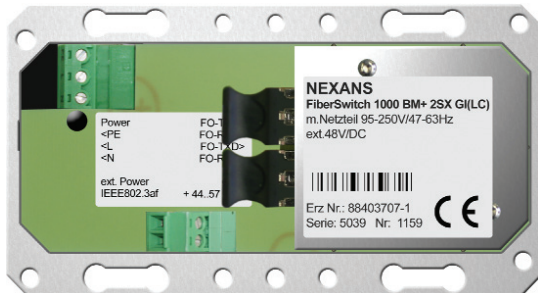
Rückansicht: FiberSwitch 1000 BM+ 2SX G(LC) Basismodul
